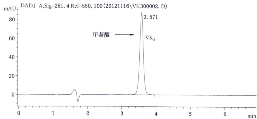
图 B.1 甲萘醌标准溶液(浓度为 5 \mu\text{g/mL} )色谱图
